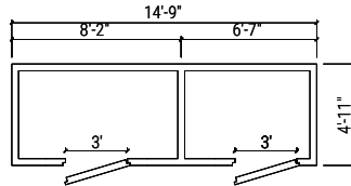
CMB5X15-8C7F-36R36CR
