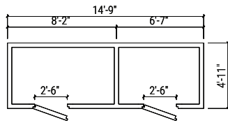
CMB5X15-8C7F-30L30L
