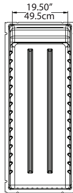
6025XL Interior
